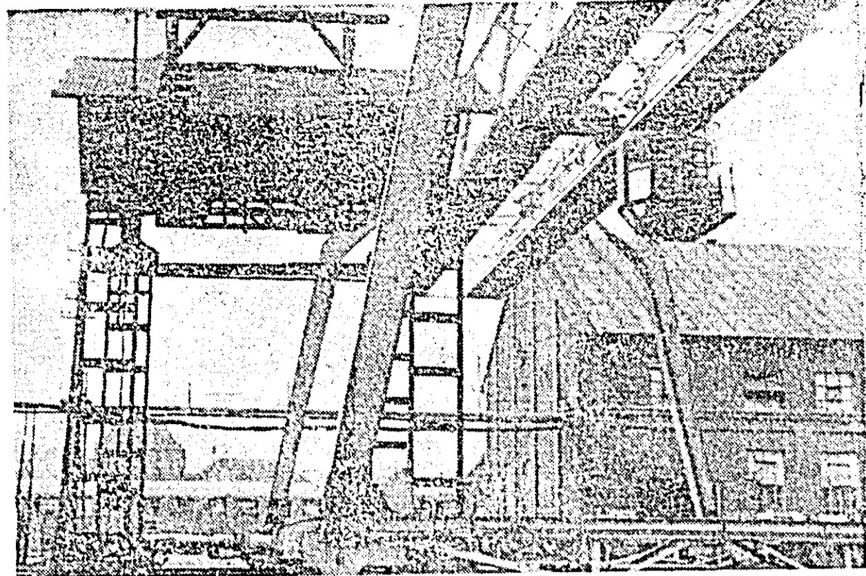
ÎN CLISEU: Noua macara de 5 tone. Instalată la sectorul II al Uzinelor de vagoane
