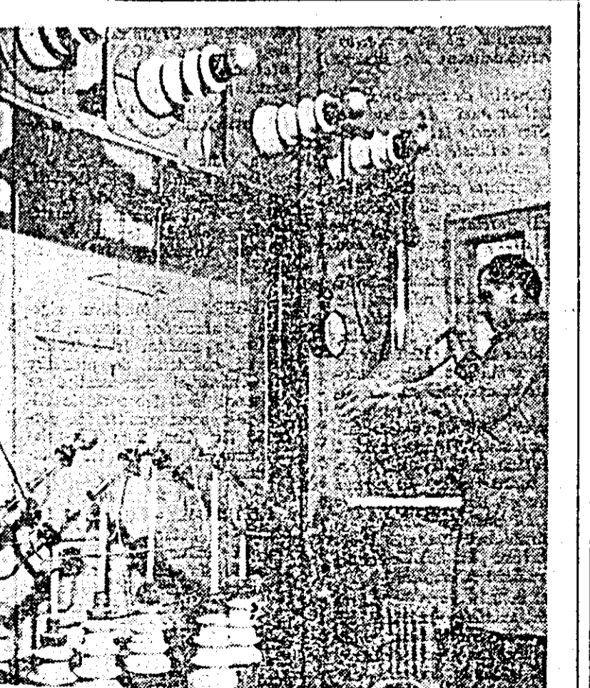
Aspect de la Institutul de Iglenă și protecția muncii din București. Ing. Ion Enciu — șeful laboratorului de electrosecuritate pregătind instalația de înaltă tensiune, în vederea încercărilor la străpungere a echipamentelor electrolizante folosite ca mijloace individuale de protecție la instalațiile electrice.
