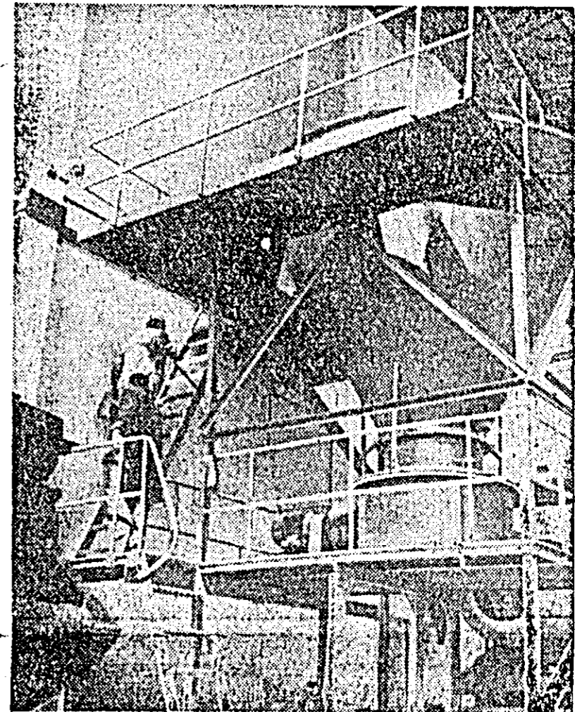
Turnătorii Uzinei de strunguri trece printr-o continuă înnoire și modernizare a utilajelor. În ultimul timp la dispoziția turnătorilor a fost pusă și această stație modernă pentru preparat nisip. Stația respectivă cernă și usucă nisipul și dezbate pămîntul de turnare.
