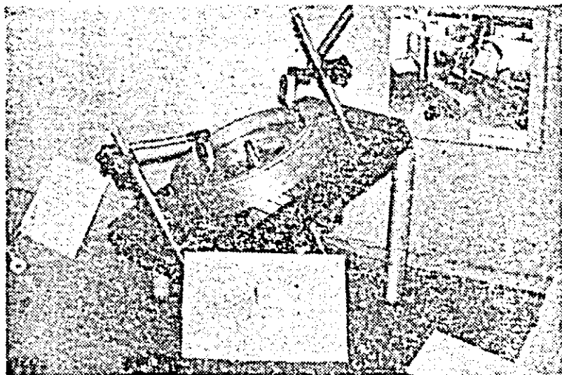
La Întreprinderea de strunguri, activitatea de căutare a noului dobîndește nota permanenței. ÎN IMAGINE: un dispozitiv de verificare radială și frontală a batajelor prin a cărui folosire productivitatea muncii în operația de control crește cu 50 la sută.
