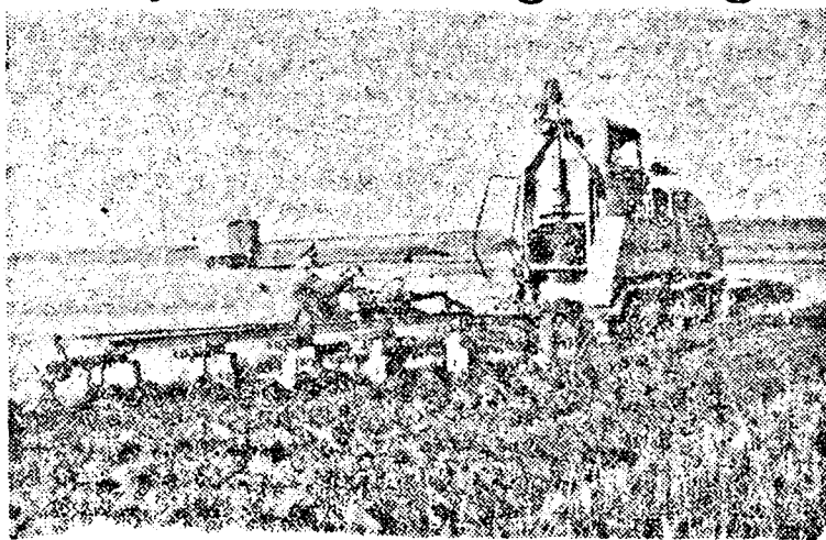
A szovjet gépkonstruktőrök nagyszerű gépet alkottak: a villamosraktort, amelyet kitűnő eredményekkel használ a szocialista mezőgazdaság. A Szovjetunióban villamos gép- és traktorállomások létesítettek.
