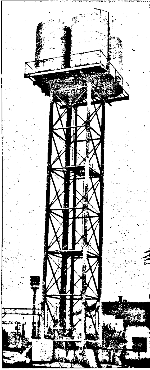
34 m înălțime, patru rezervoare metalice a 50 m.c. fiecare, iată câteva din caracteristicile tehnice ale castelului de apă construit în premieră pe țară, în întregime pe structură de rezistență metalică, de către Mont Star SRL în gara Curtici. Foto: VIOREL MUSCA
