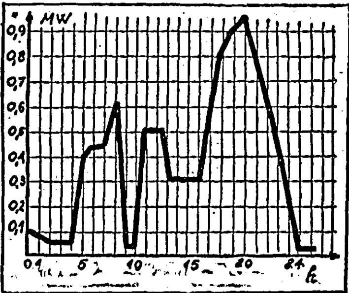
Curba consumului pe o zi la balastiera Ghioroc a I.E.I.A.M.C.
