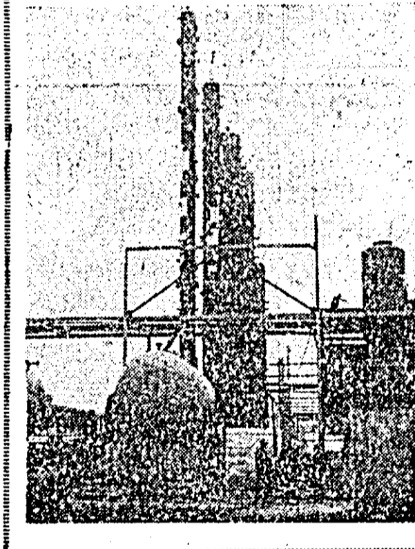
Combinatul petrochimic din Pitești va realiza începînd din anul 1968 aproape 80 la sută din producția țării de etilenă și peste 70 la sută din cea de propilenă. ÎN FOTOGRAFIE: Secția de aromate și hidrogenare din cadrul complexului de piroliză.
