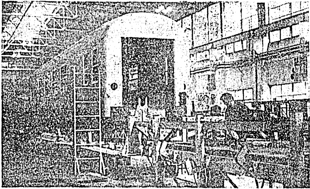
Uzina de vagoane, Sectorul II. În această hală, dată în exploatare anul trecut, se assemblează vagonul suburban. Pînă acum constructorii arădeni au dat peste prevederi 4 asemenea vagoane. În foto: un instantaneu de muncă.
