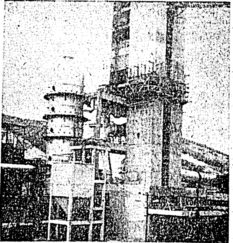
Vedere parțială a modernelor fabrici de dolomită din Zlațiș.
