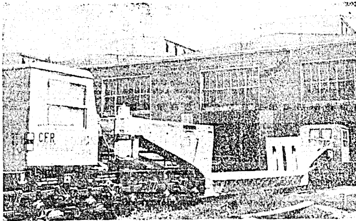
Între alte produse realizate în acest an la Uzinele de vagoane a fost și un lot de vagoane pe 10 osii, cu platformă scundată, pentru transportul unor piese grele pînă la 140 tone. Proiectanții au avut în vedere între altele caracteristicile tehnice și reducerea consumului de metal.
