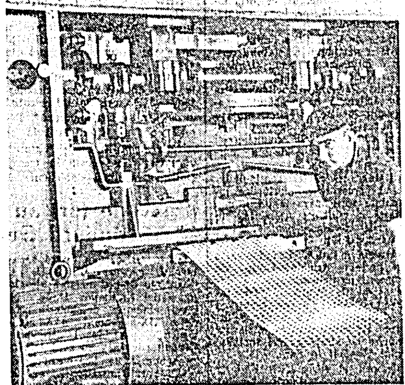
Pentru a asigura bunul mers al producției și creșterea continuă a productivității muncii, la Uzinele de vagoane s-au construit cu forțe proprii diferite utilaje speciale. Printre acestea se numără și mașina de expandat tablă.
