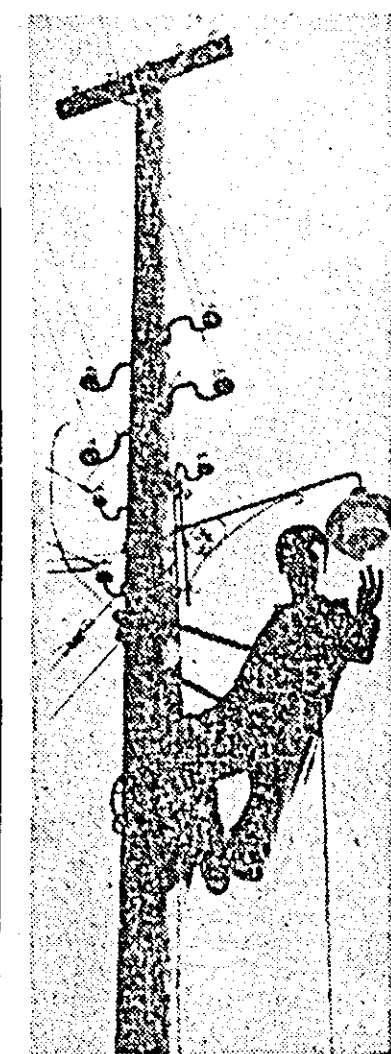
Colectivul de muncă al șantierului iluminat public de la Uzina electrică a întreprins în acest an numeroase lucrări de extindere și modernizare a iluminatului public din orașul nostru. Printre lucrările recent pu- se sub tensiune se numără ex- tinderea iluminatului public cu un kilometru pe 10 străzi din cartierul Grădiște și montarea celor 16 corpuri de iluminat cu vapori de mercur pe malul Mu- reșului.
