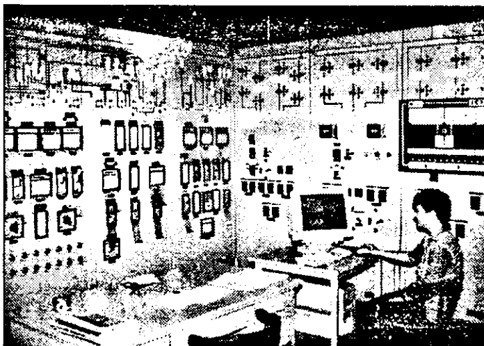
Pupitrul de comandă, asistat de calculator, al instalației de difuzie-purificare.
