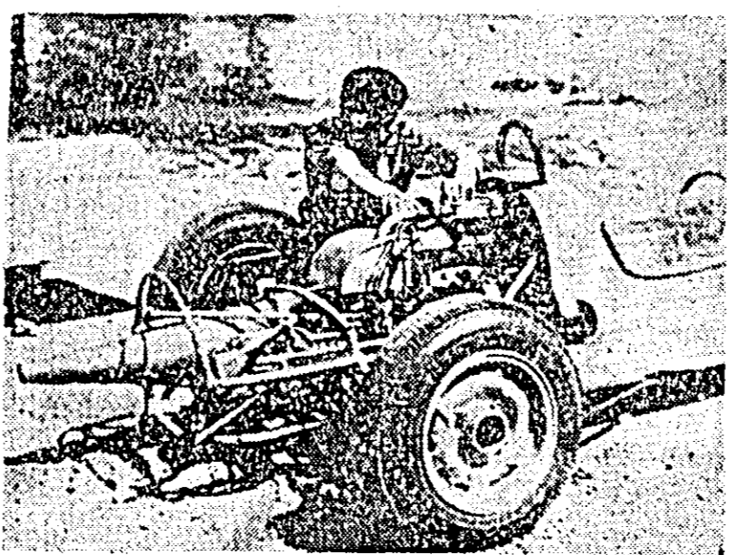
R. S. CEHOSLOVACA. — Membri ai Automotoclubului Interprinderii Dukla din Habarov, (vestul Boemiei), conduci de constructorul Otakar Hamal, au realizat un automobil de curse de tip „F-3”. Corpul automobilului este din foi metalice (laminat). Viteza maximă atinsă în cursa de probă a fost de 160 kilometri pe oră.
