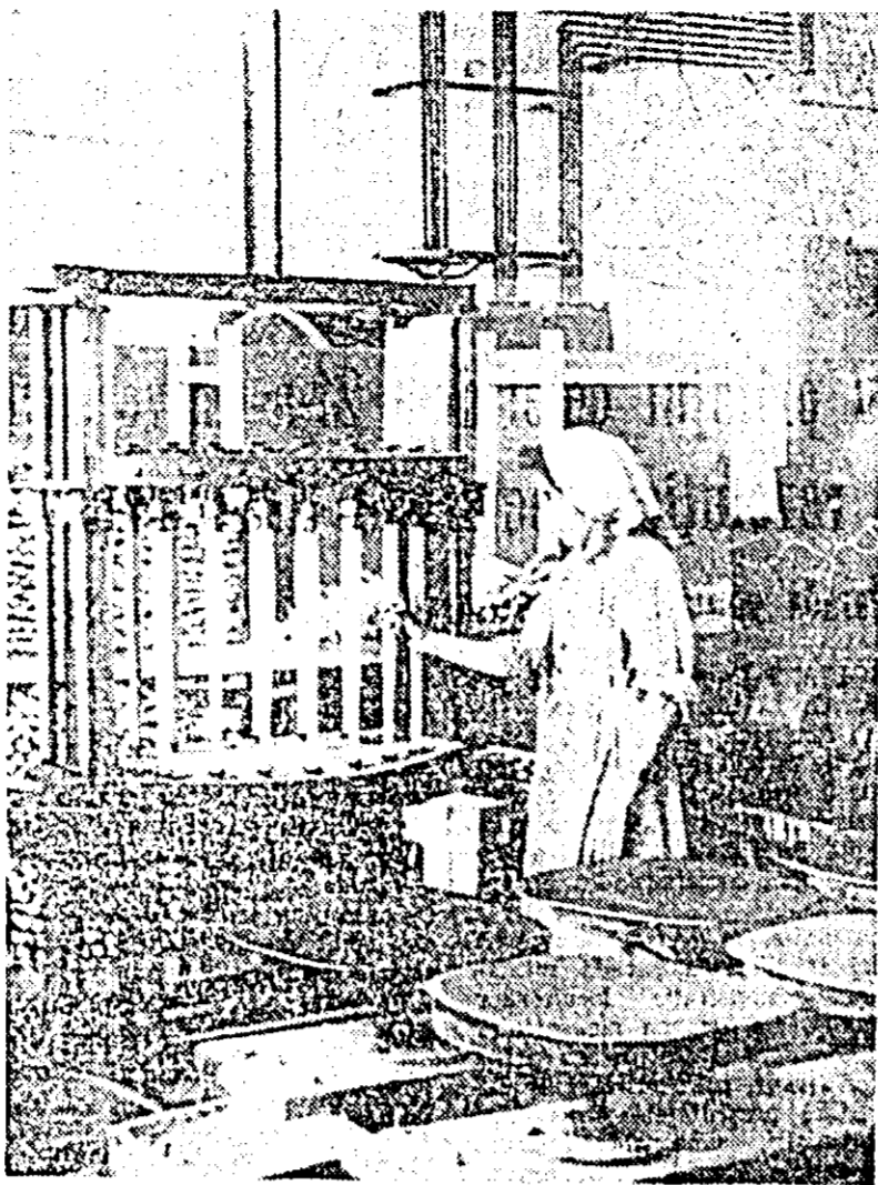
La fabrica de mobilă curbată „Răsăritul” din Pincota mecanizarea unor operații manuale aduce o contribuție importantă la obținerea unei productivități sporite, la îmbunătățirea calității produselor. Rezultate superioare se obțin și cu ajutorul acestei mașini prin care s-a mecanizat operația de șlefuit și grindare a picioarelor de scaune.
