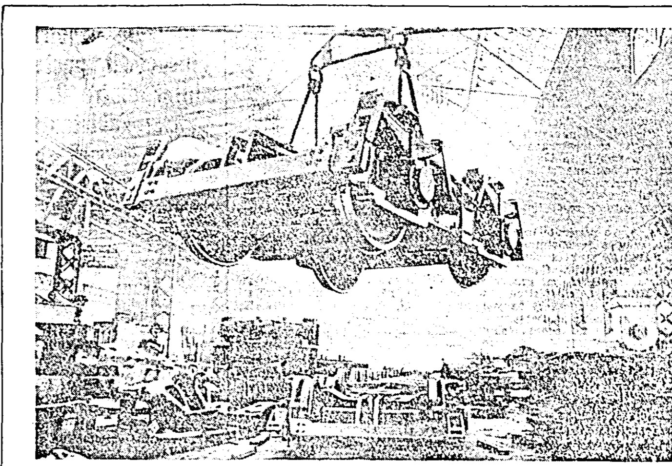
Aspect de la uzinele „Gh. Dimitrov”. Se montează boghiul unui vagon.
