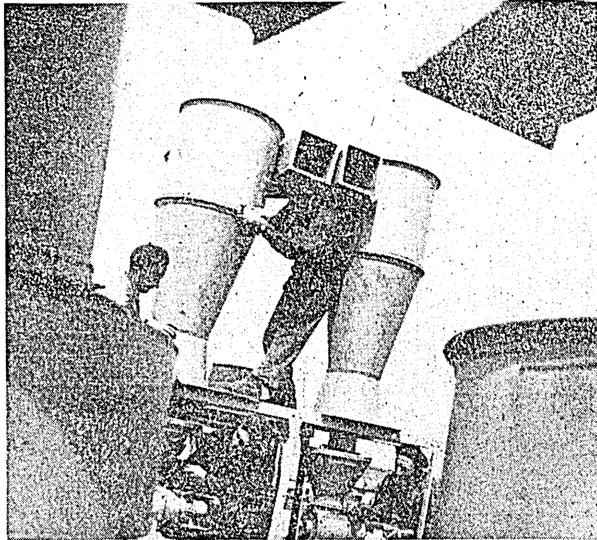
În atelierul de lăcătușerie din cadrul sectorului 4 al Uzinei de reparații, condus de tovarășul Nicolae Timaru, se execută în prezent o serie de utilaje și instalații pentru agricultură. IN CLIȘEU: Șeful de echipă Liviu Oarga și lăcătușii Anton Kitzinger, Andrei Bacoș și Mitru Ștef, executând montajul general al bateriei de praf pentru morile de cînoace de 5 tone.
