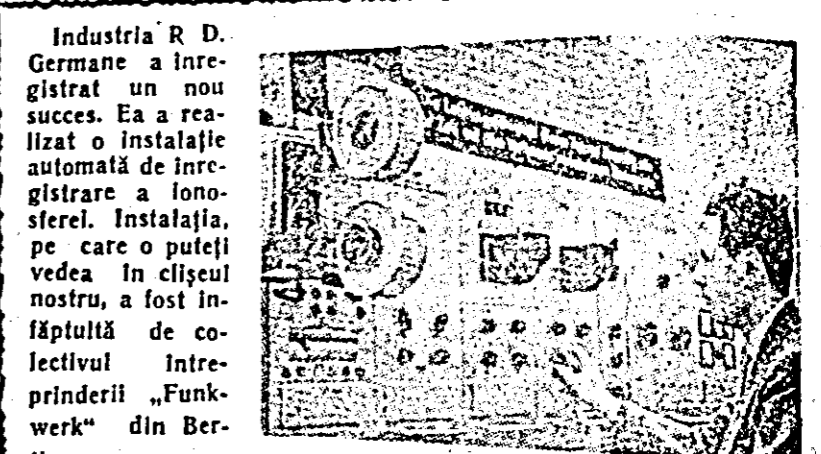
Industria R. D. Germane a înregistrat un nou succes. Ea a realizat o instalație automată de înregistrare a fonosferei. Instalația, pe care o puteți vedea în cliseul nostru, a fost înfăptuită de colectivul întreprinderii „Funkwerk” din Berlin.
