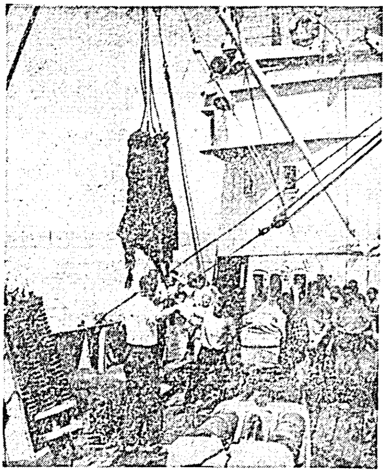
Această dragă a ajuns la o adâncime de câteva mii de metri. Ea a scos la suprafață mostre de roci de bază de pe fundul Oceanului Indian.
