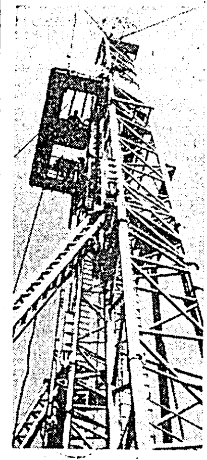
Instalația românească de foraj LD instalată recent pe teritoriul Poloniei — votevodatul Kielce.
