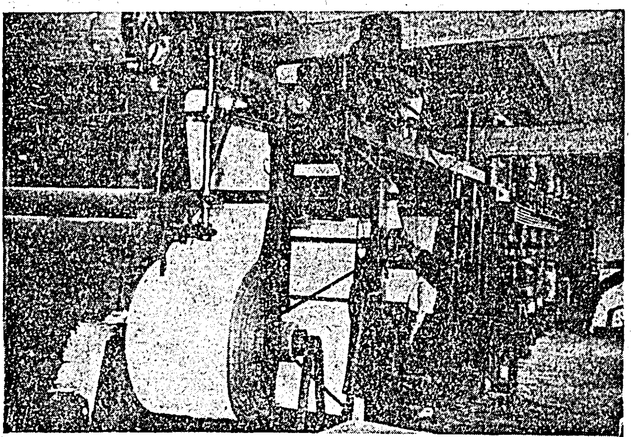
În vopsitoria fabricii „Teba” se aplică procedeul de împregnare la rece cu coloranți reactivi care dau un colorit viu și frumos țesăturilor. După rularea concomitentă cu împregnarea, țesătura se face uscarea, materialul staționează 2-15 ore pe role, acoperit, pentru a se produce procesele chimice de difuzie și fixare.
