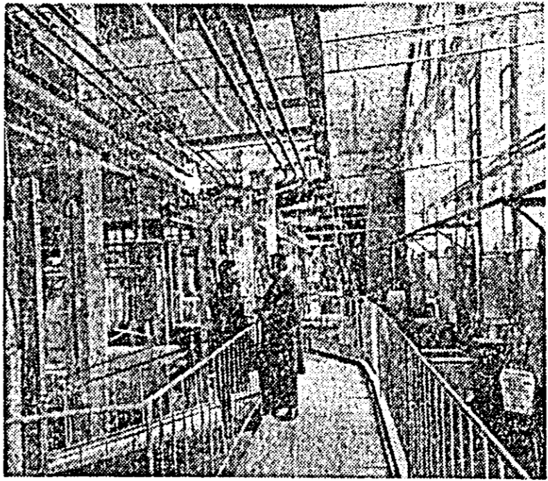
Fabrica de sticlă Azuga, execută articole de ambalaje, borcane și butelii de sticlă. Clăusele reprezintă un aspect de ansamblu al liniei tehnologice de alimentare a cuptoarelor de topit sticlă.
