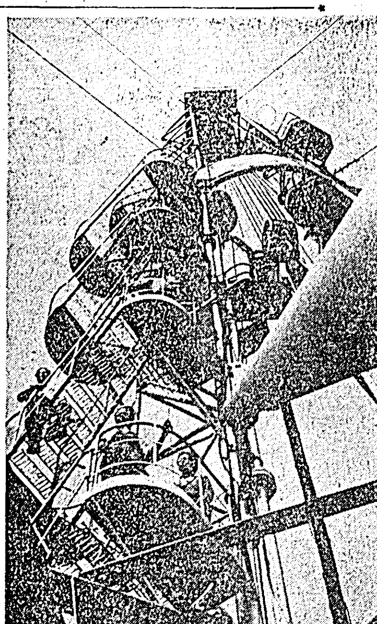
O nouă instalație sovietică de înaltă productivitate pentru forajul cu turbidă sau rotor.
