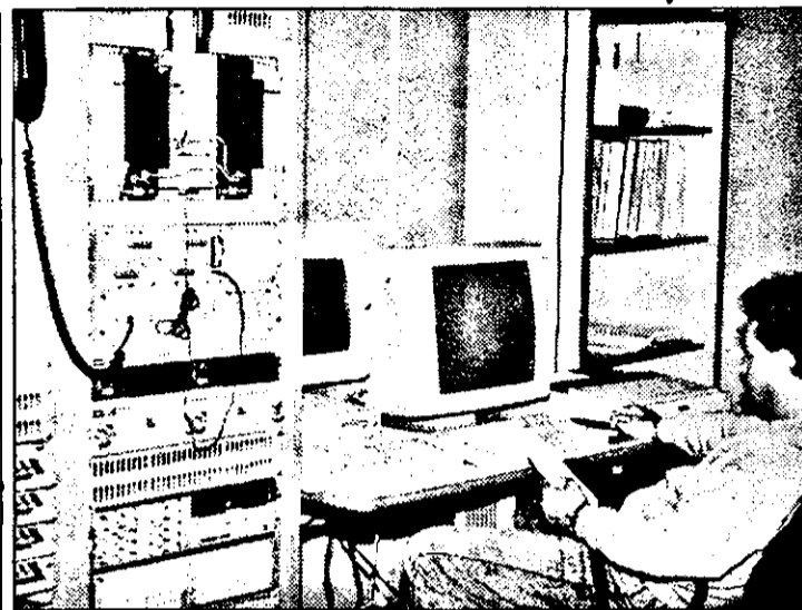
Echipamentele din sala tehnică asigură legătura cu capul radar de la Mânăstur, cât și cu aeronavele aflate în zbor.
