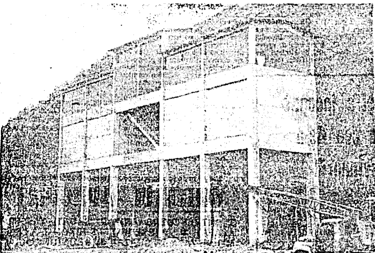
Pe valea Mureșului, la cariera din Bătuța, a început în cincinalul trecut, construcția unei moderne stații de concasare, care asigură un însemnat spor de producție, un înalt grad de mecanizare a operațiilor de extragere și prelucrare a pietrei. Noua stație va face ca producția carierei să sporească cu cca 14.000 tone piatră anual.
