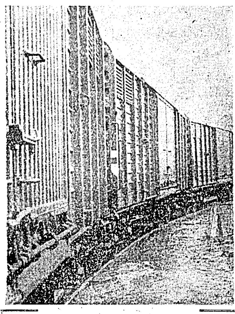
Vagoane marfă pe patru osii cu o capacitate de 80 tone, construite din metal, cu caracteristici și parametri la nivelul tehnicii actuale. Aceste vagoane se construiesc în serie la Uzinele de vagoane Arad.
