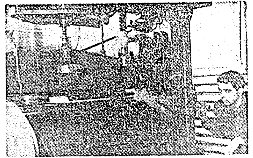
Uzinele Ștefan Ghergar de la sectorul II al Uzinelor de vagoane lucrează la mașina de expandat tablă. El se evidențiază prin calitatea lucrărilor și prin depășirea sarcinilor de plan.
