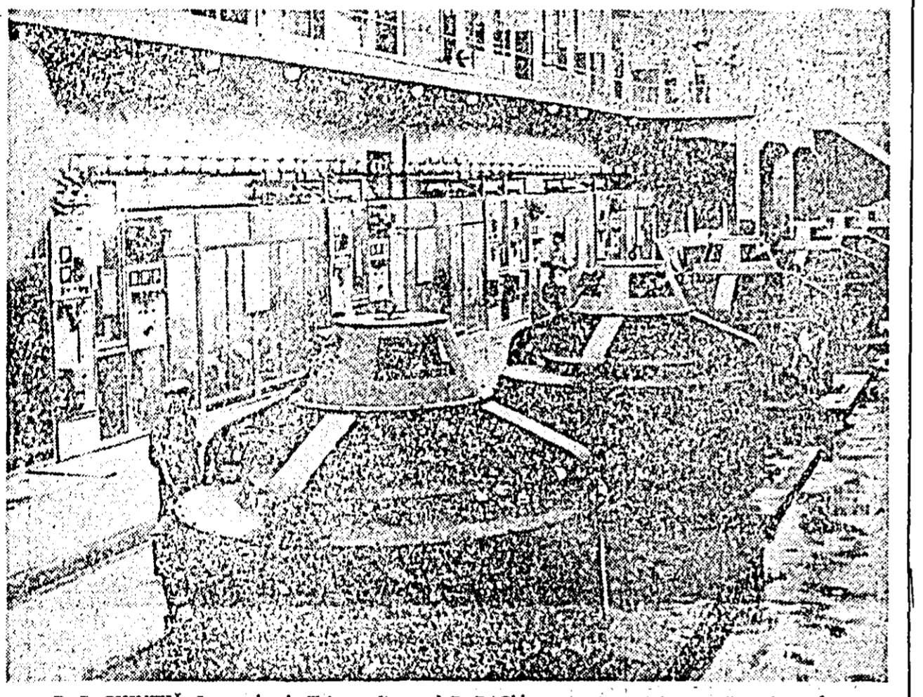
R. P. CHINEZĂ. În provincia Tzansu din estul R. P. Chineze s-a construit o nouă stațiune electrică prin pompare care asigură irigația a 42.000 de hectare de ore șarii și drenarea unor imense terenuri din această provincie.
