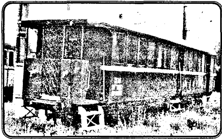
Vagonul remorcă nr. 1, construit de Uzina de vagoane Arad în anul 1906, pentru calea ferată Arad-Podgoria și reconstruit, de curând, în aceleași ateliere.
