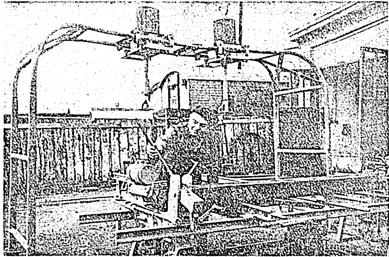
Inovatorul Izidor Dalcă de la atelierul L.R. CFR a realizat pînă acum 12 inovații. Ultima sa inovație este mașina pentru reparat traverse. Înaltă, această muncă se execută manual. Cu ajutorul mașinii, productivitatea muncii crește considerabil, iar calitatea reparațiilor va fi mai bună.
