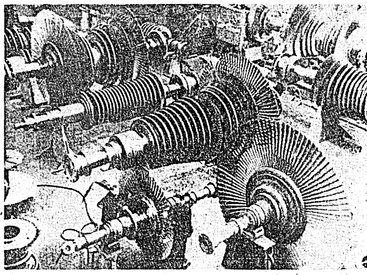
U.R.S.S.: Uzina de produse metalice din Leningrad — sectorul de asamblare a puternicilor turbine cu abur.
