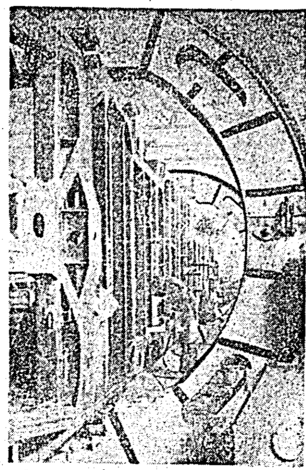
Sectorul II al întreprinderii de vagoane. În imagine: dispozitiv rotativ pentru sudaj șastul vagonului de călători.
