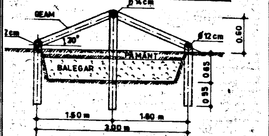
Răsadniță cu două pante îngropate
