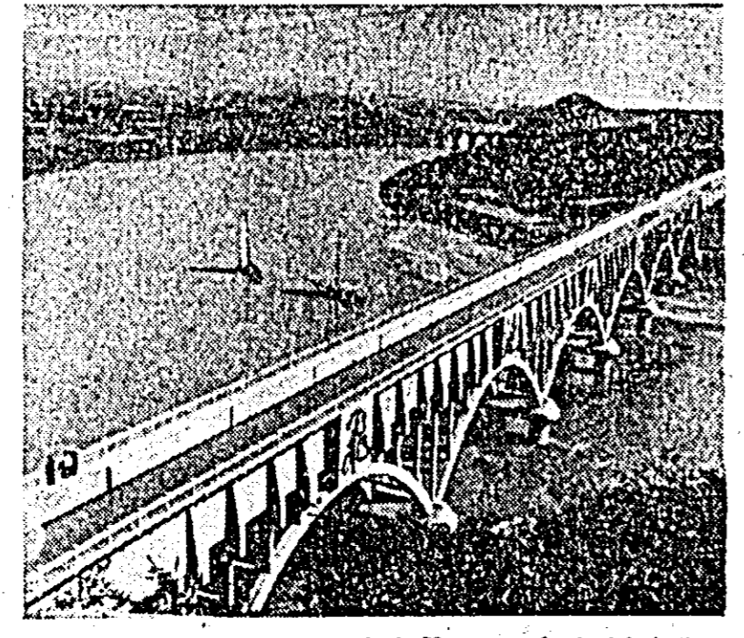
În China centrală, în provincia Hunan s-a dat în folosință un nou sistem de irigație. În imagine, conducta de apă de la Chechin lungă de 530 metri, care face parte din sistemul de irigație Shaosan și traversează rîul Licenului.
