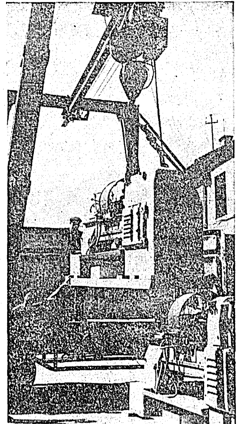
Uzina de strunguri. La rampa de încărcare un nou lot de strunguri este pregătit pentru expediere.
