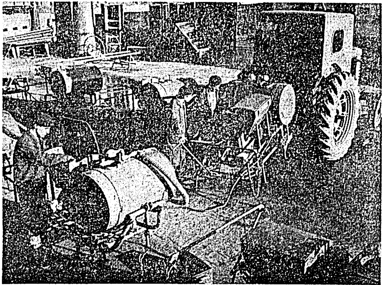
Fabrica de ventilatoare București. Se fac probele la un lot de mașini de stropit și prăfuit.
