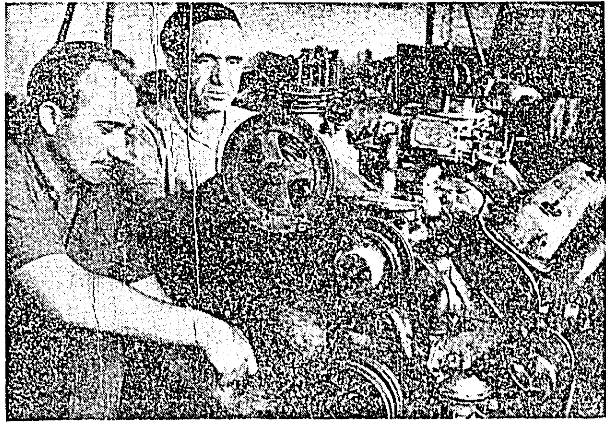
În atelierul mecanic al întreprinderii comunale Arad lucrează și tovarășii Alexandru Titizer și Ioan Bota. Reparațiile efectuate de ei sînt întotdeauna de bună calitate. IN CLIȘEU: cei doi muncitori făcînd ultima revizie la un motor de autobuz pe care l-au reparat.
