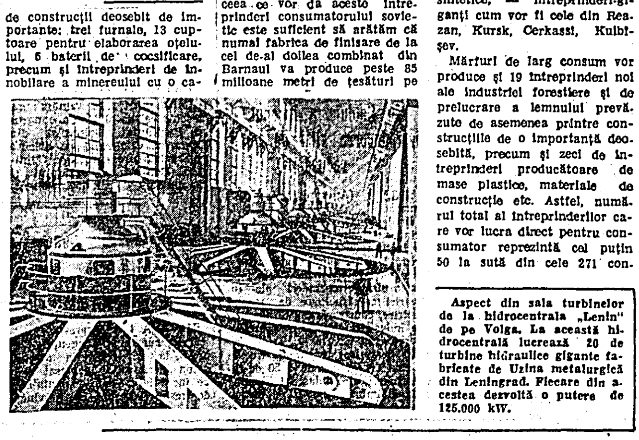
Aspect din sala turbinelor de la hidrocentrala „Lenin” de pe Volga. La această hidrocentrală lucrează 20 de turbine hidraulice gigante fabricate de Uzina metalurgică din Leningrad. Fiecare din acestea dezvoltă o putere de 125.000 kW.
