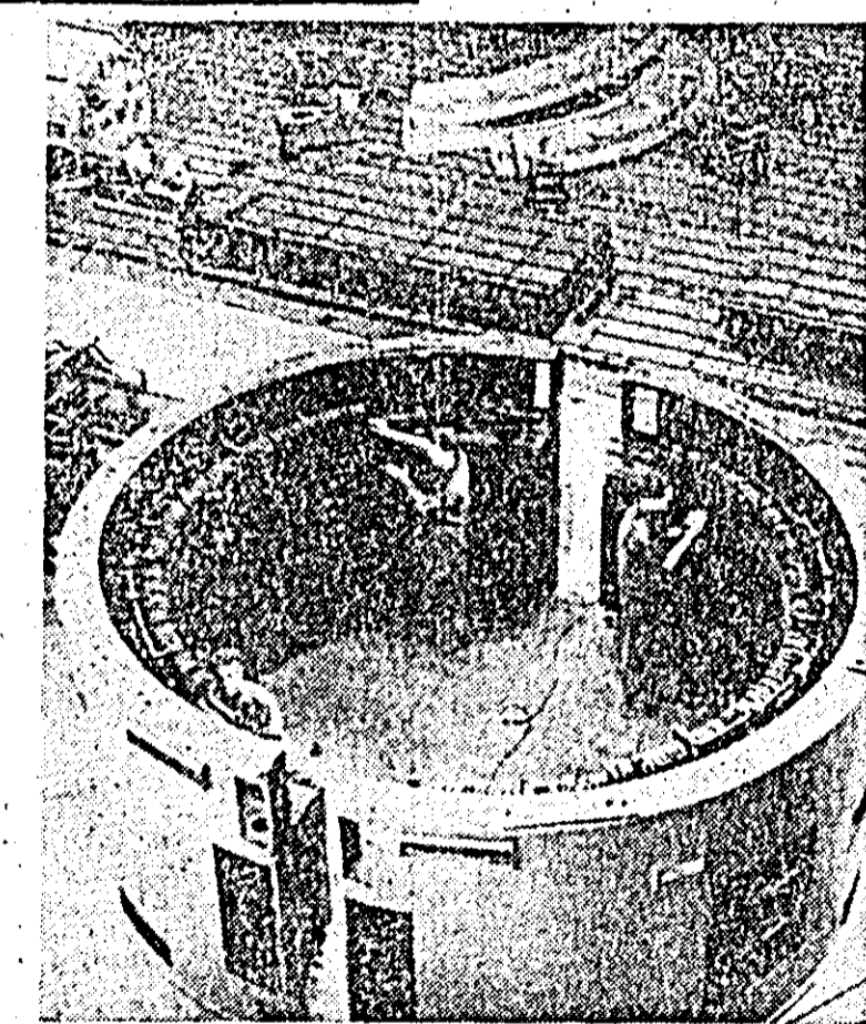
La secția utilajele electrice a Uzinei constructoare de mașini din Reșița se lucrează la construirea unui motor pentru turbină de 7,5 megawati.
